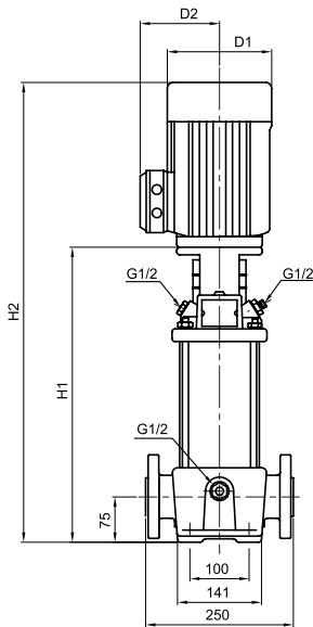
Flange(DIN-ANSI-JIS) PN 25 / DN25/32
