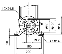
Flange(DIN-ANSI-JIS) PN 25 / DN25/32
